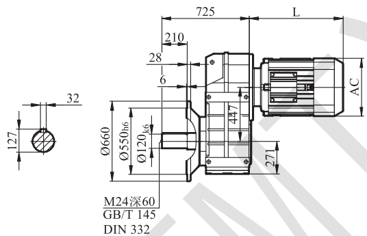
GFF157
