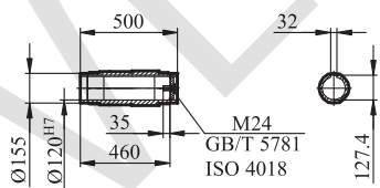
GFA/GFAZ/GFAF157输出轴
