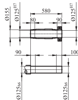
GFH/GFHZ/GFHF157输出轴
